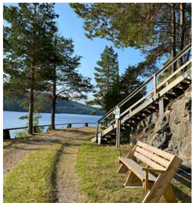
Geopark Indalsälven: Vid Stadsberget finns berg i dagen som vittnar om jordens utveckling och skyltar som förklarar. Foto: Carina Landin
